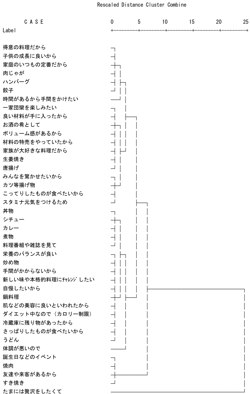
別添図表VI-7 クラスタ分析のデンドログラム
